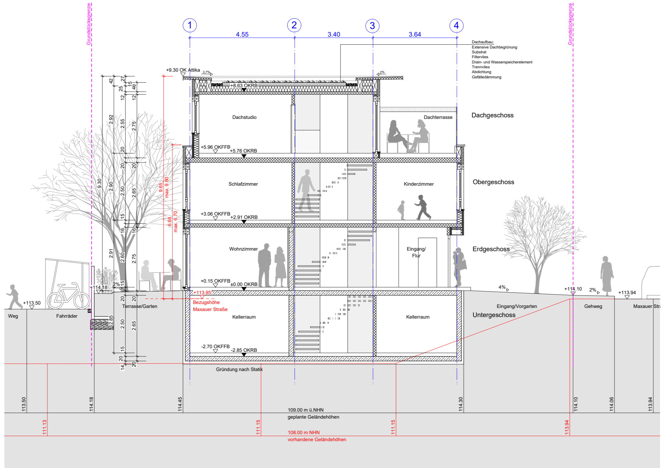
Schnitt B-B Großer und kleiner Typ
