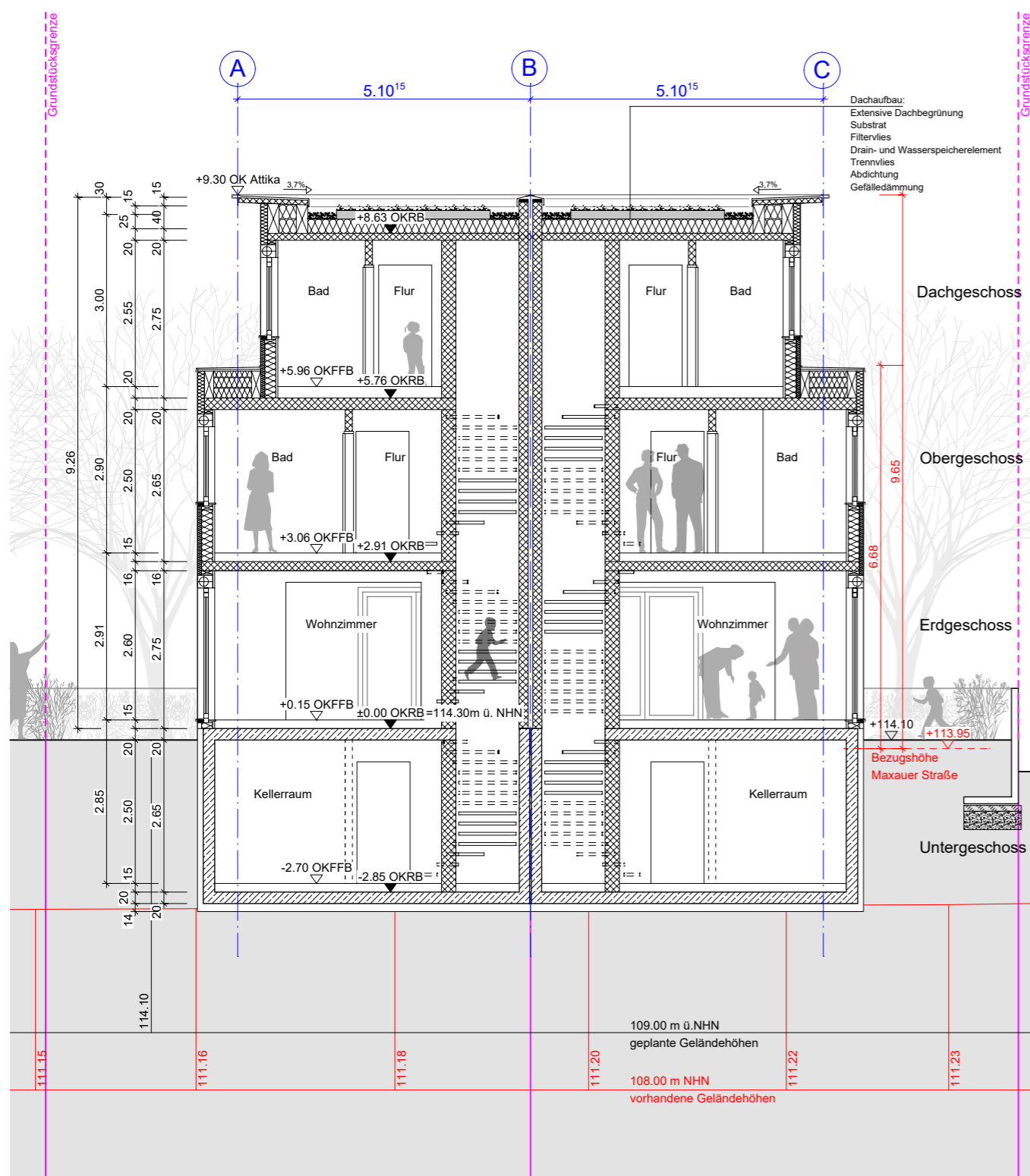
Schnitt A-A Kleiner Typ
