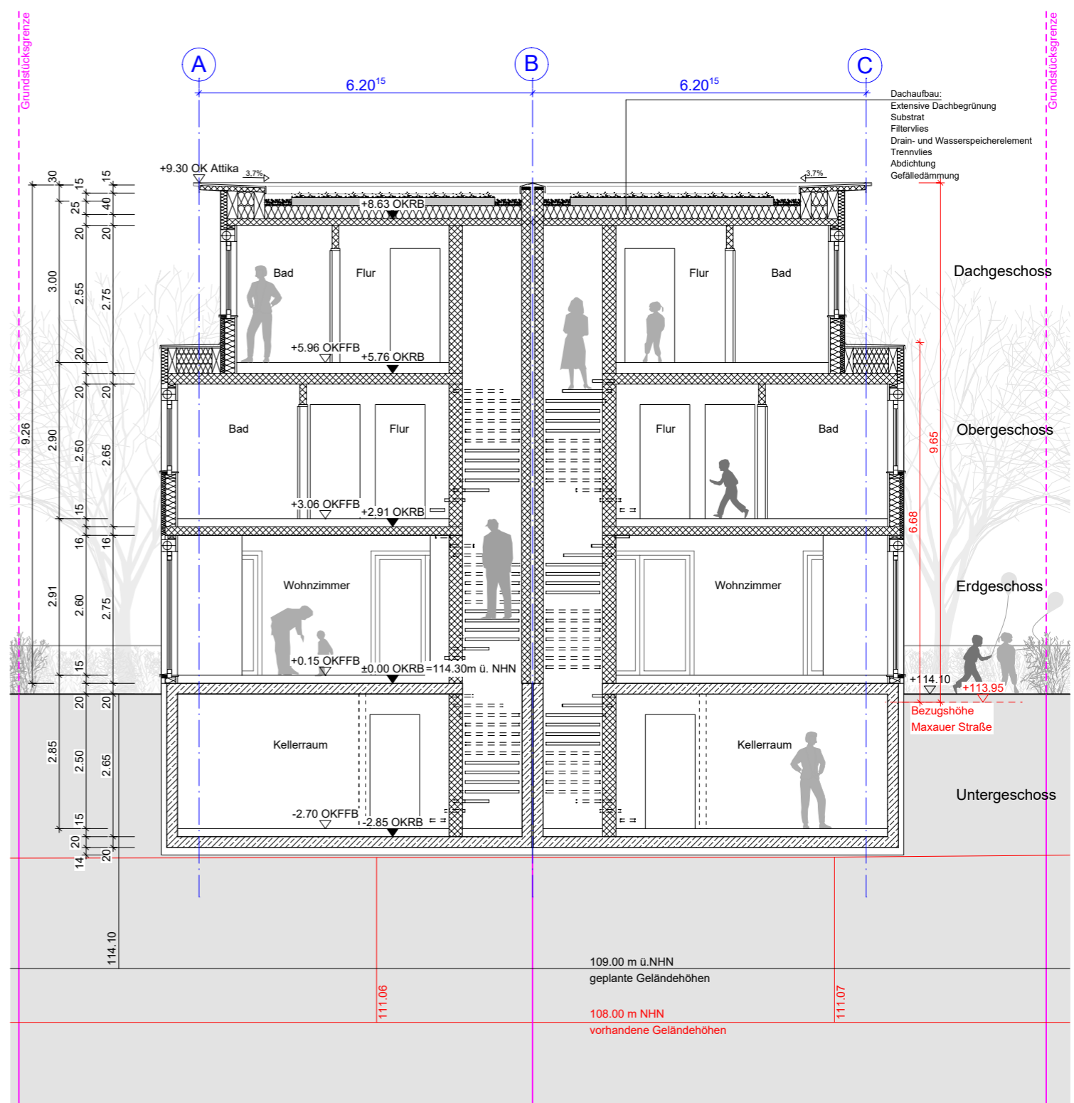
Schnitt A-A Großer Typ
