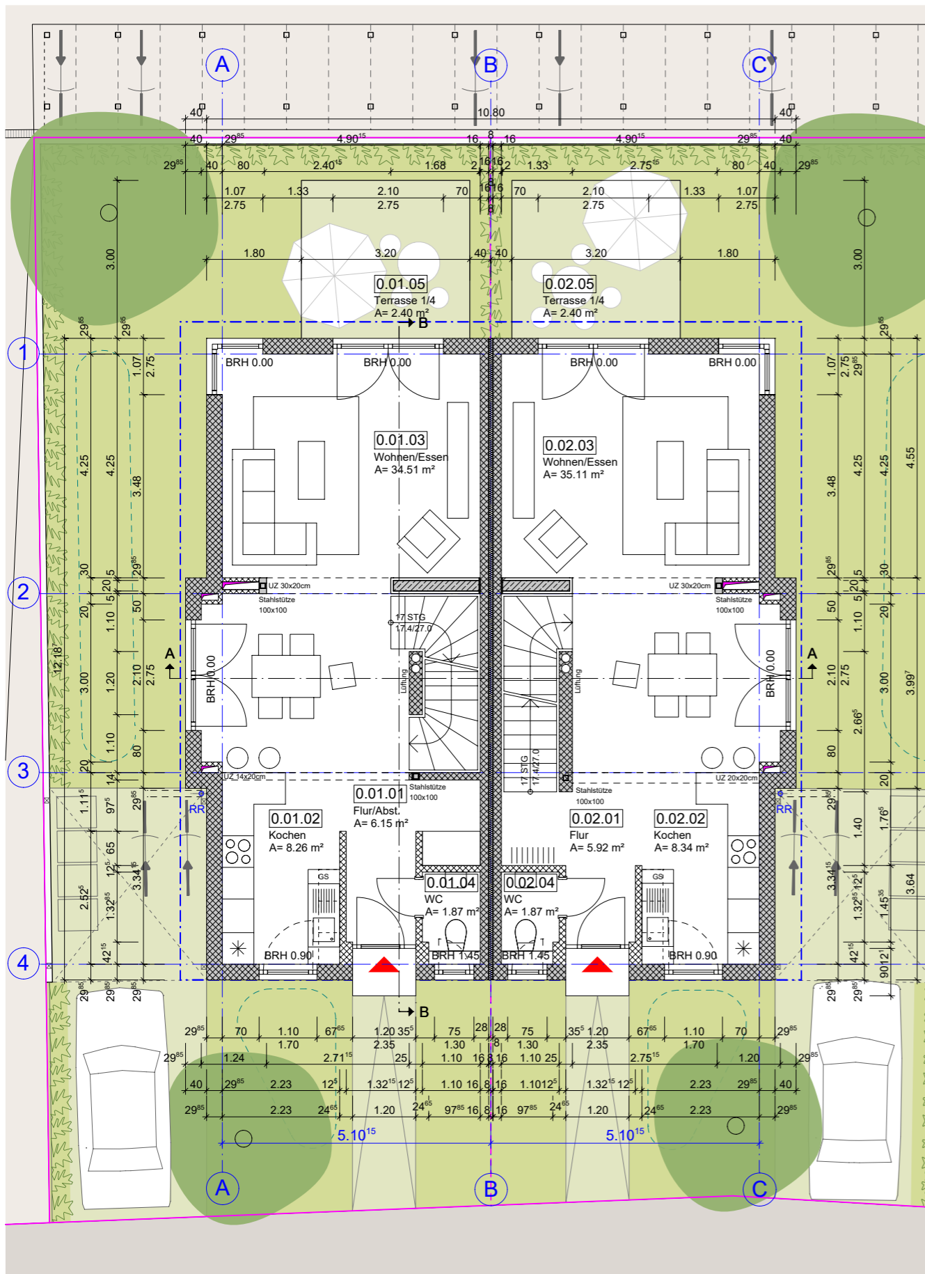
Grundriss Erdgeschoss Kleiner Typ
