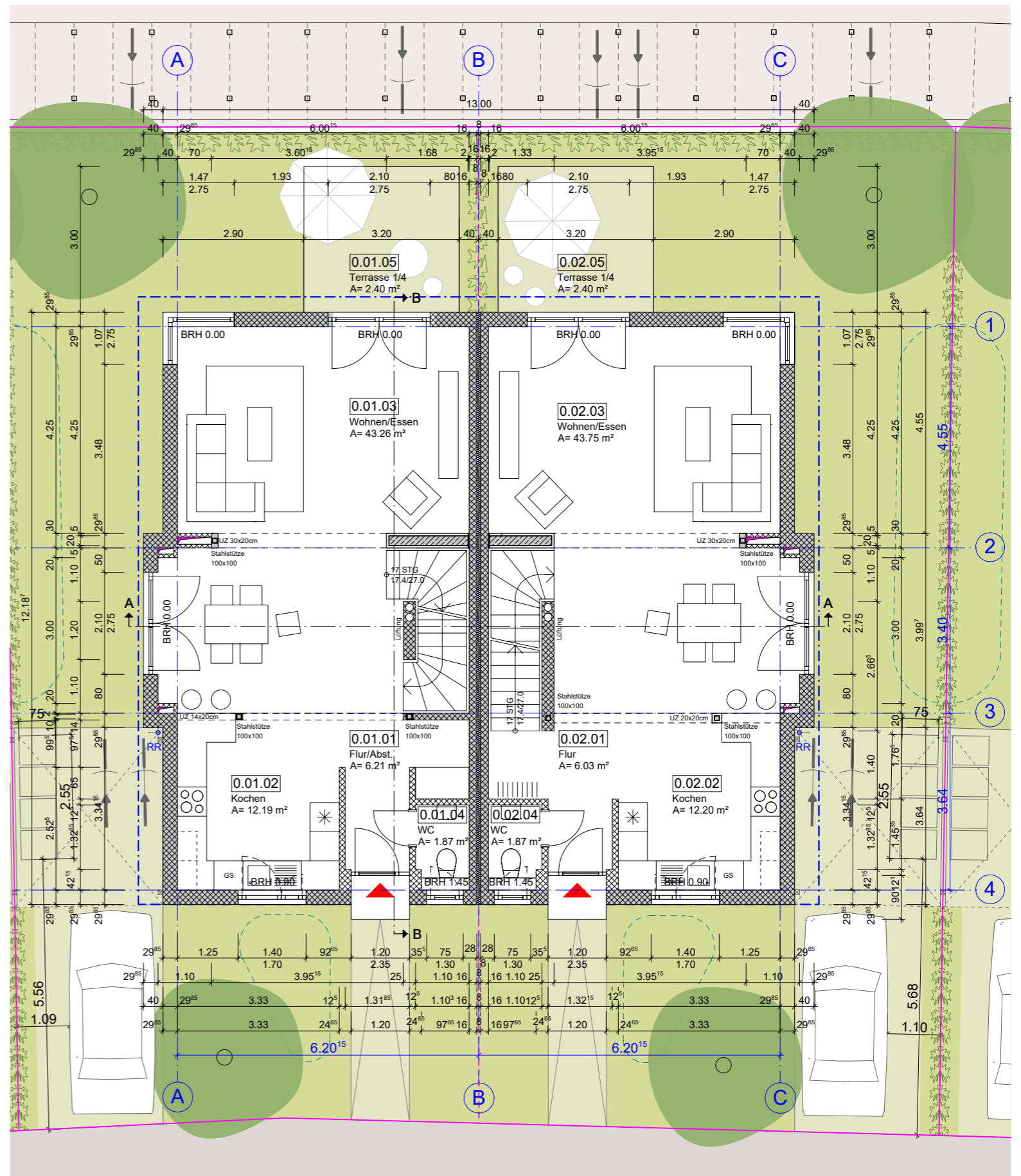
Grundriss Erdgeschoss Großer Typ
