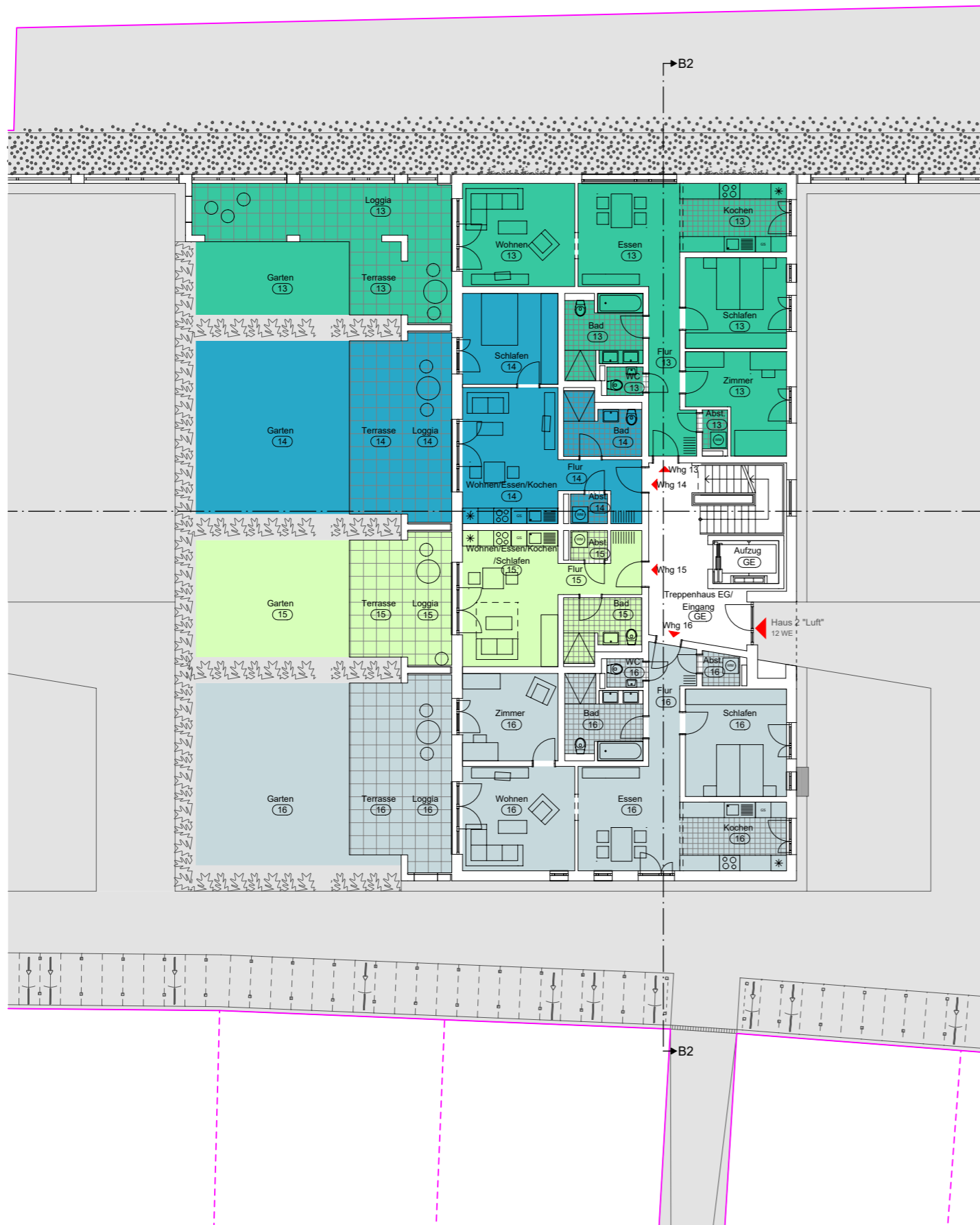
Erdgeschoss
